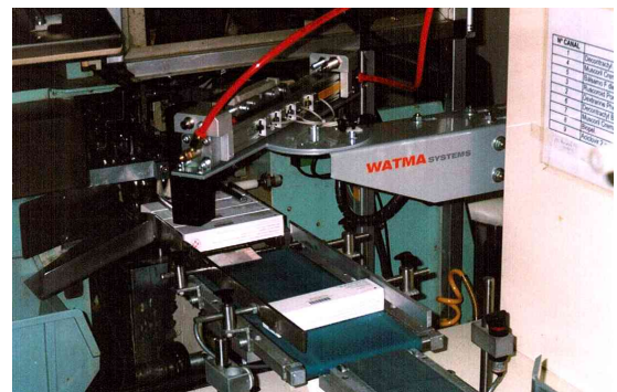
Detalle del movedor integrado en la línea de producción. Vista delantera.
